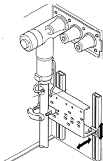
Kabelschaltfeld Kabelcel
