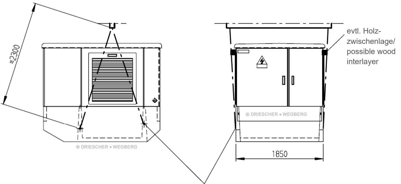
Trichterseilösen / funnel rope loops RD30x3,5
