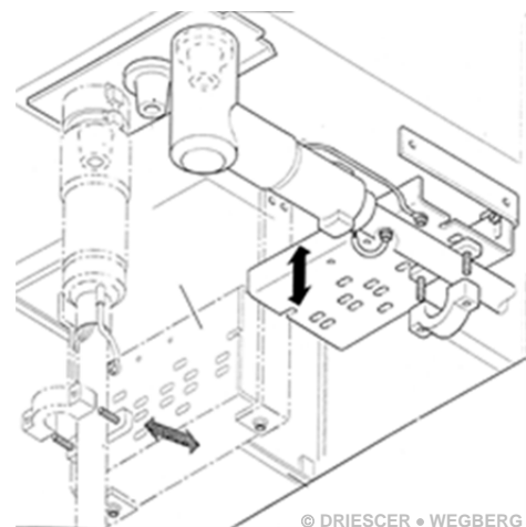
Trafoschaltfeld Transformer cubicle
