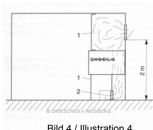
Bild 4 / Illustration 4
