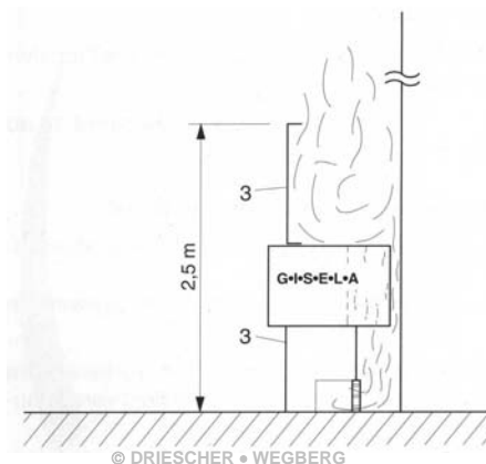
Bild 5 / Illustration 5
